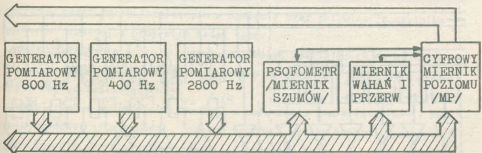
Rys. 5. Elementy Bloku Pomiarowego
