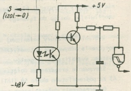
Rys. 3b. Układ oddzielający sygnały z UD
