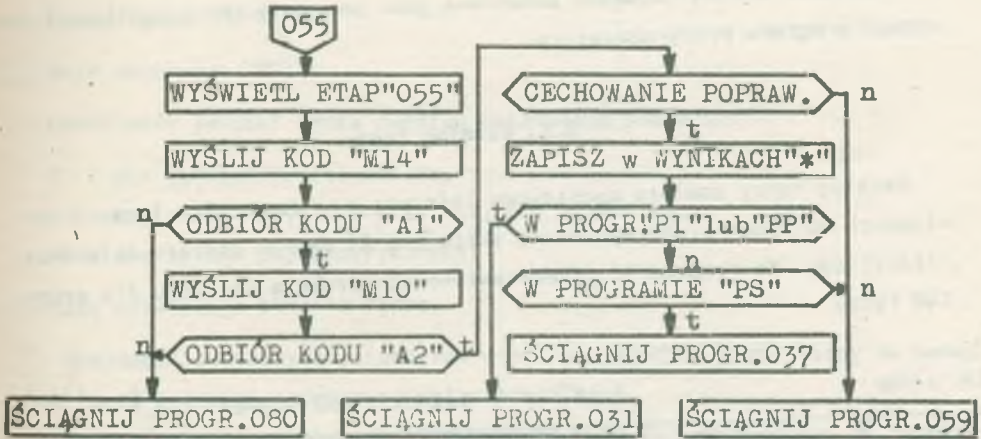
Rys. 10. Przykładowy algorytm etapu pomiarów łączy /ETAP 055 "zakończenie cechowania mierników"/
