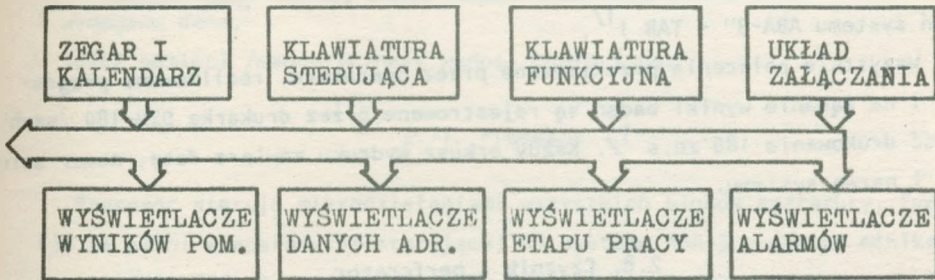
Rys. 7. Elementy tablicy manipulacyjnej aparatury A3
