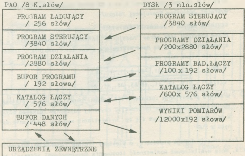
Rys. 9. Obszary pamięci aparatury sterującej A3
