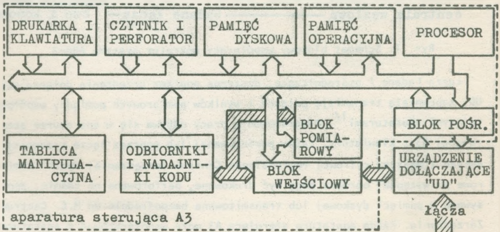
Rys. 2. Schemat blokowy aparatury sterującej A3 systemu ABA-3
