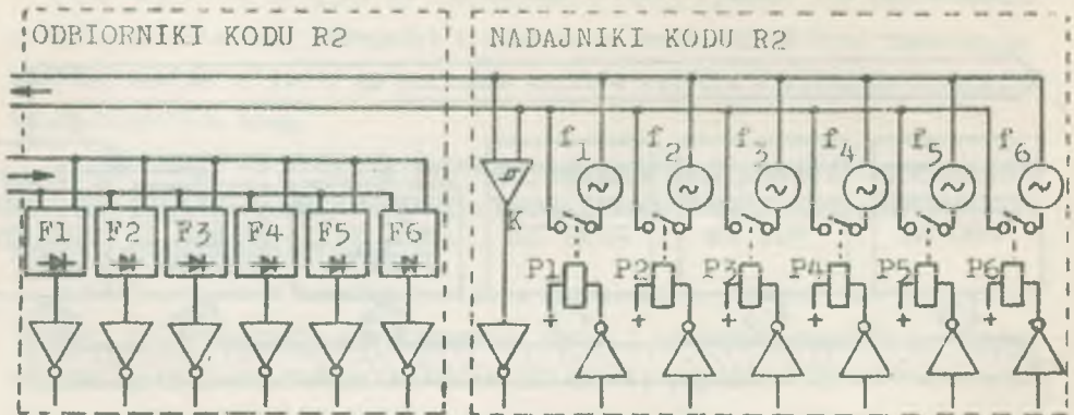
Rys. 6. Uproszczony schemat odbiorników i nadajników kodu
