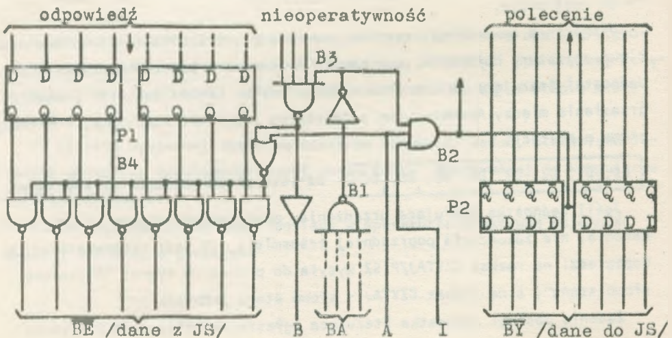
Rys. 8. Uproszczony schemat Jednostki Sterującej
