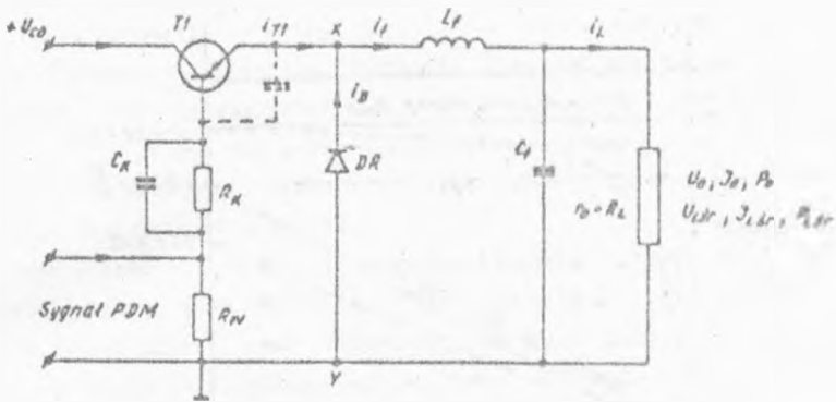
Rys. 8. Uproszczony układ tranzystorowego wzmacniacza modulującego klasy AD mcz obciążony rezystancją zastępczą R_L = r_o odpowiadającą układowi wzmacniacza modulowanego w.cz widzianemu od strony zasilania przy modulacji amplitudowej
