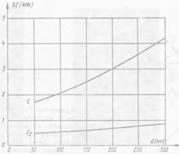
Rys. 5. Odstępny pomiędzy sąsiednimi węzłami wypadkowego natężenia pola w funkcji odległości od stacji nadawczej przy interferencji fali przyziemnej i jonosferycznej odbitej od warstwy E lub F_2
