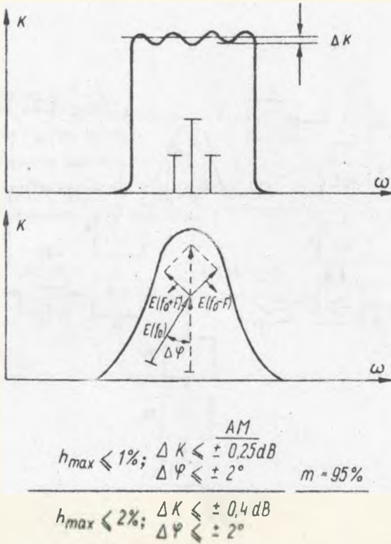
Rys. 13. Dopuszczalne tolerancje przebiegu charakterystyk przenoszenia toru transmisyjnego /tłumieniowej \Delta K i fazowo-częstotliwościowej \Delta \varphi /ze względu na zniekształcenia harmoniczne obwiedni wywołane naruszeniem wewnętrznej amplitudowo-fazowej struktury sygnału zmodulowanego
