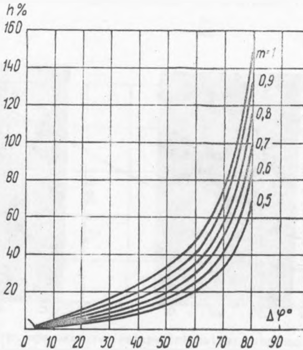
Rys. 9. Zależność zniekształceń nieliniarnych obwiedni sygnału w systemie dwuwstępowej modulacji amplitudowej od asymetrii fazowej wstęp bocznych względem fali nośnej
