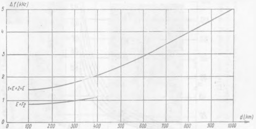
Rys. 6. Odstępny pomiędzy sąsiednimi węzłami wypadkowego natężenia pola w funkcji odległości od stacji nadawczej przy interferencji fali jonosferycznej odbitej od warstw E i F_2
