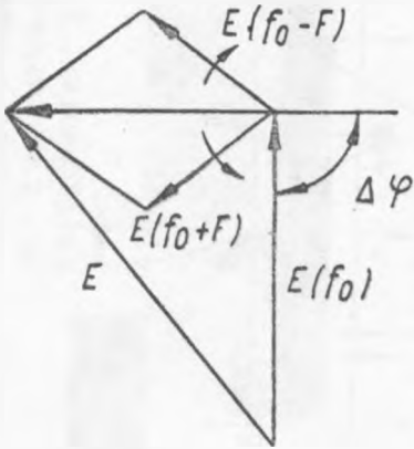
Rys. 7. Usytuowanie fazowe wstęp bocznych modulacji względem fali nośnej przy występowaniu zniekształceń fazowych grupy falowej sygnału zmodulowanego w systemie dwuwstępowej modulacji amplitudowej
