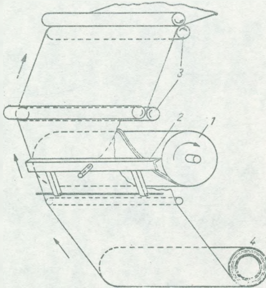
Rys. 10. Zasada zastosowania spirali przestrzennej do rozwinięcia płaskiego w odbiorniku telekopijowym
