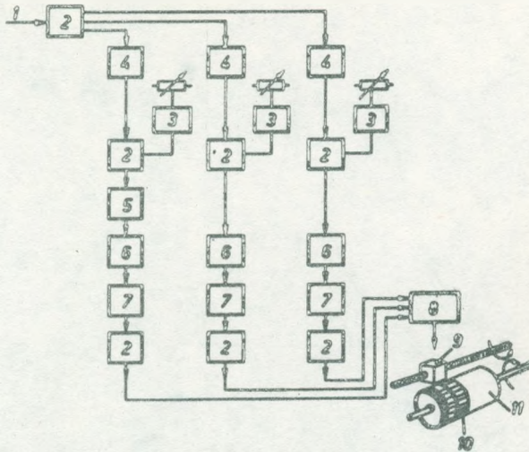
Rys. 36. Schemat blokowy odbiornika telekopti kolorowej
