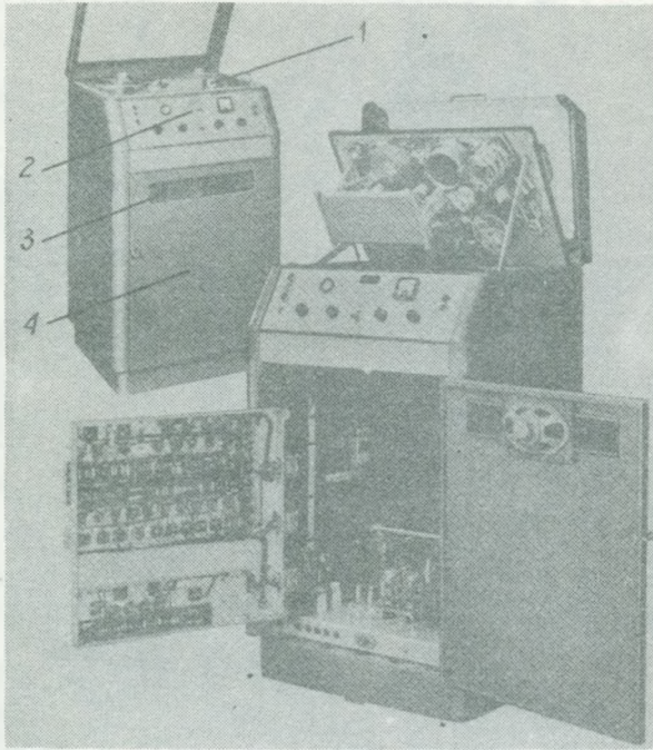
Rys. 30. Urządzenie do rejestracji na taśmie magnetycznej sygnałów telegrafii faksymilowej / wykonanie firmy Muirhead, typ D-944/
