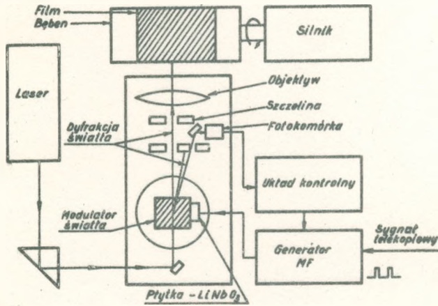
Rys. 38. Schemat blokowy układu laboratoryjnego odbiornika telekopiowego z zapisem laserowym
