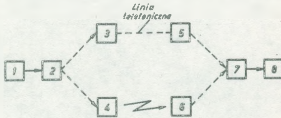
Rys. 37. Układ blokowy systemu transmisji telekoptowej przy zastosowaniu metody kodowania cyfrowego
