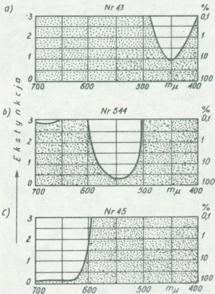
Rys. 34. Charakterystyki filtrów: ekstynkcja w funkcji długości fali /ekstynkcja-logarytm dziesiętny przepuszczalności filtru barwnego, selektywnego/: a/ filtr „niebieski”, b/ filtr zielony, c/ filtr „czerwony”
