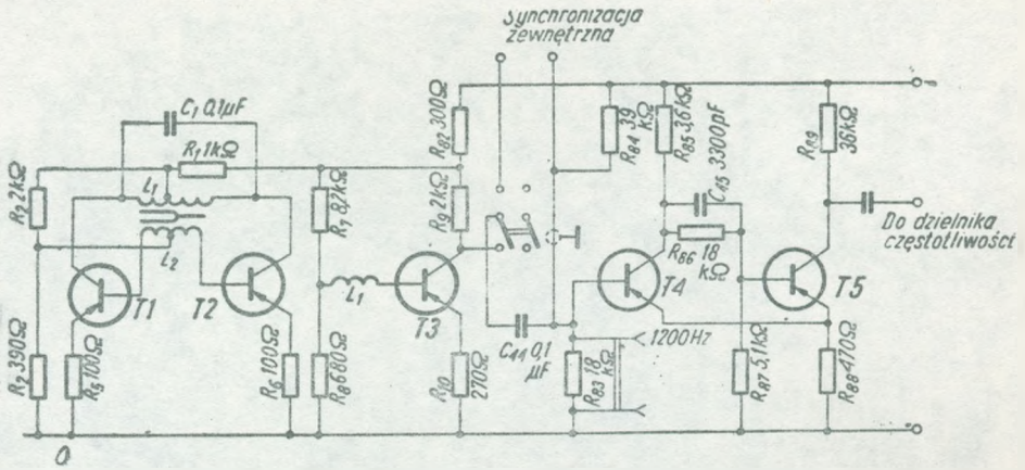
Rys. 9. Fragment schematu zasadniczego nadajnika telekopii czarno-białej, typ FAK-D / ZSRR/
