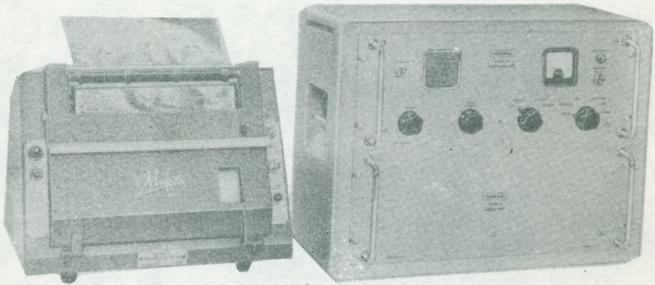
Rys. 29. Widok aparatu telekopii odcieniowej firmy Muirhead, typ D-900-S/1 "Satellite facsimile receiver"
