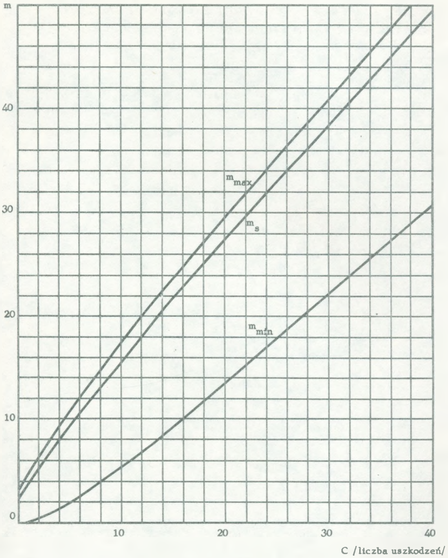
Rys. 7. Wykres pozwalający określić intensywności uszkodzeń i granice przedziałów ufności
