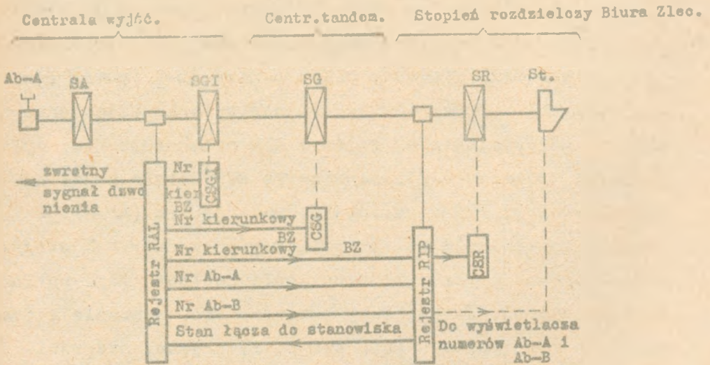
Rys.4. Połączenie wewnętrzstrefowe między dwoma abonentami
