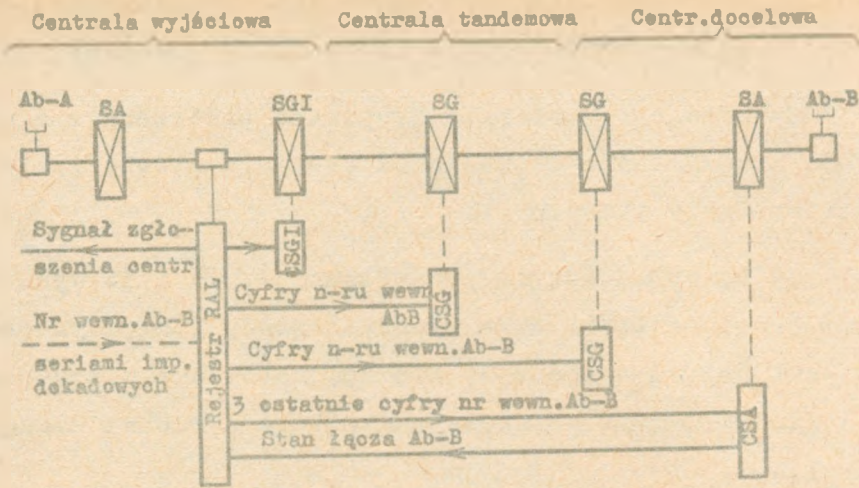
Rys.4. Połączenie wewnętrzstrefowe między dwoma abonentami
