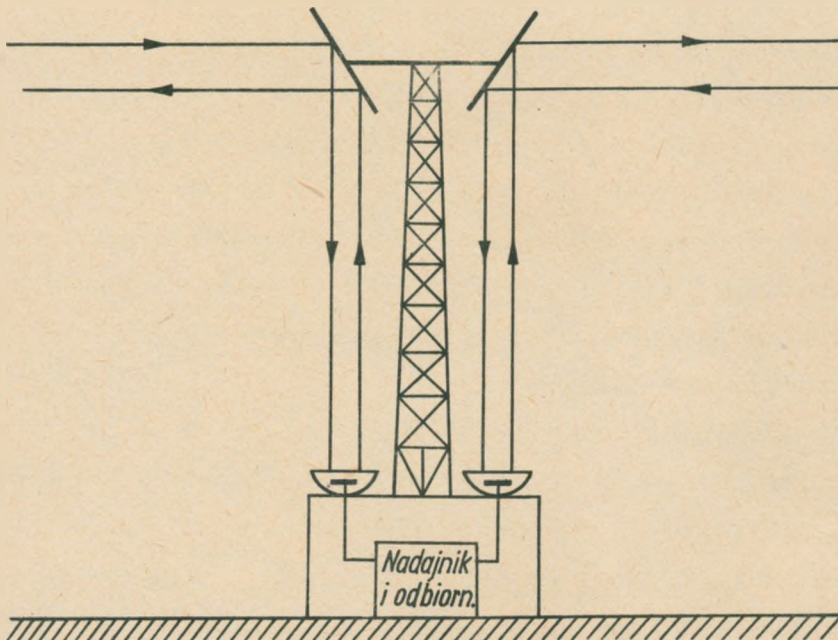
Rys. 12. Kierunkowe odpromieniowywanie energii za pomocą płaskich reflektorów
