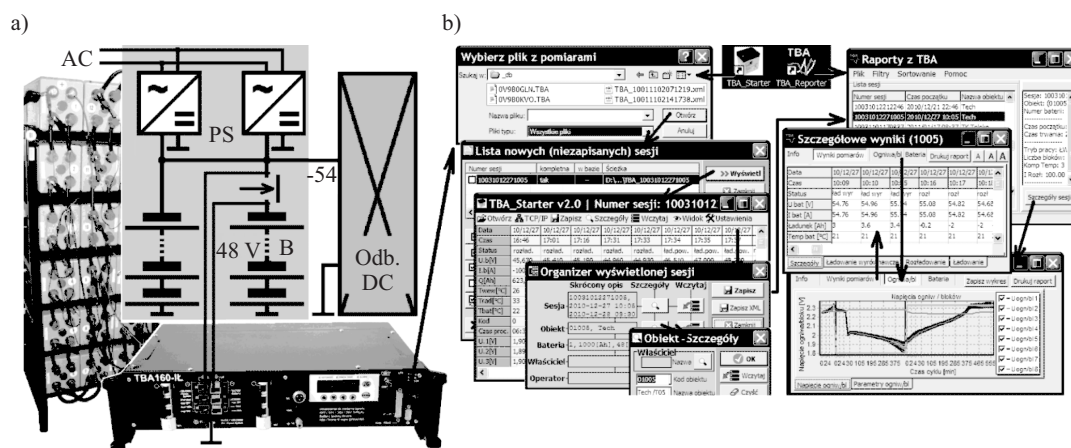
Rys. 4. Badanie baterii akumulatorów urządzeniem TBA160-IL (a) i pełne wyniki badań (b)
