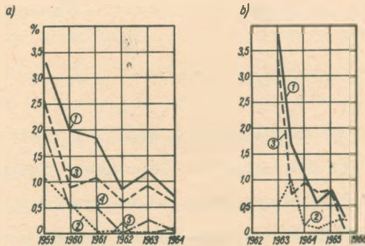
Rys. 1. Graficzne przedstawienie analizy przerw w pracy linii radiowej: a/ wyniki pomiarów przeprowadzonych w NRD [3], b/ wyniki pomiarów przeprowadzonych w IŁ
