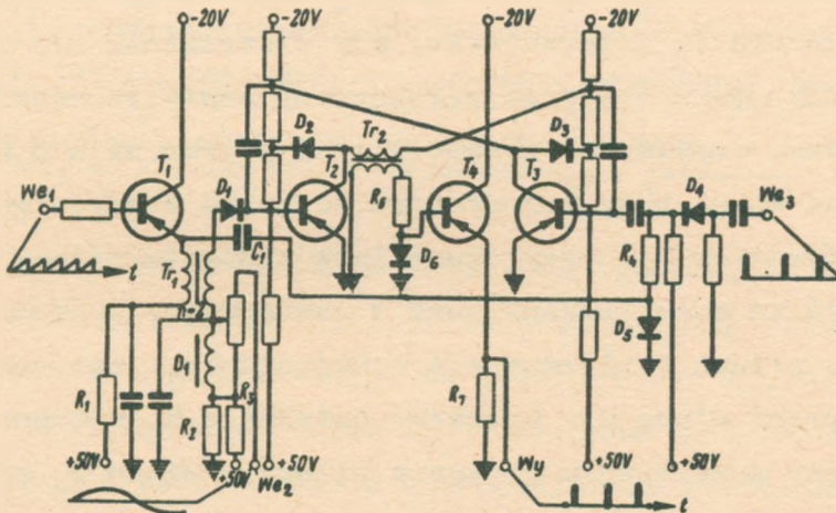
Rys. 13. Modulator kanałowy linii radiowej UR24
