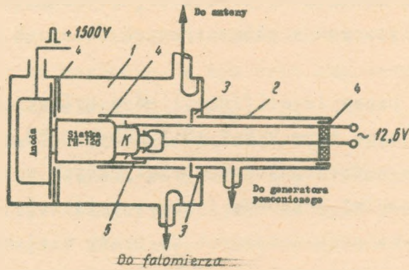
Rys. 5. Uproszczony schemat ideowy generatora nadajnika
