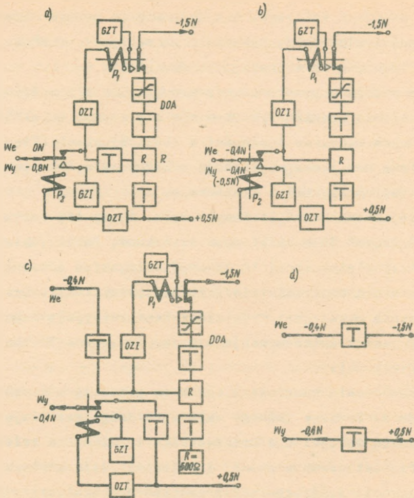
Rys. 22. Schemat blokowy zakończenia m.c.s. w różnych układach pracy: a) układ jednotorowy końcowy, b) układ jednotorowy bez tłumika, c) układ dwutorowy z translacją sewu indukcyjnego, d) układ dwutorowy z retranslacją sewu tonowego
