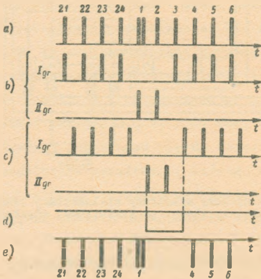
Rys. 19. Zasada "gaszenia" impulsów kanałów odgałęzionych
