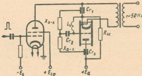
Rys. 6. Schemat ideowy generatora i manipulatora
