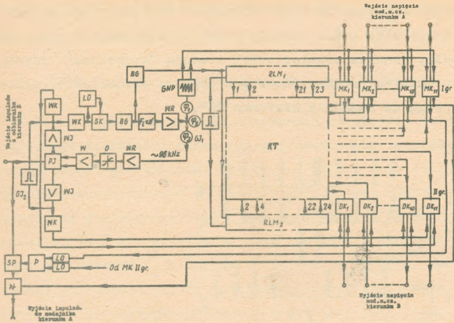
Rys. 18. Uproszczony schemat blokowy aparatury wielokrotnej linii radiowej UR124 pracującej w układzie stacji przekąźnikowej odgałęźnej
