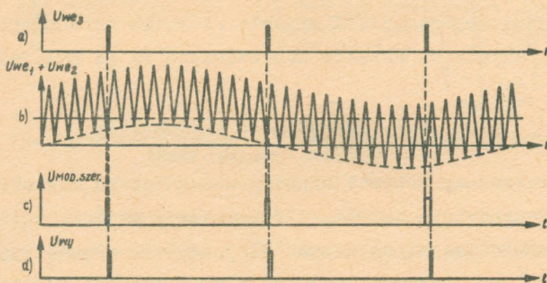
Rys. 14. Oscylogramy przebiegów napięć w modulatorze kanałowym a) impulsy o f_p = 8 kHz, b) napięcie piłkowe o f = 96 kHz nałożone na napięcie modulujące, c) impulsy modulowane w szerokości, d) impulsy wyjściowe modulowane w położeniu
