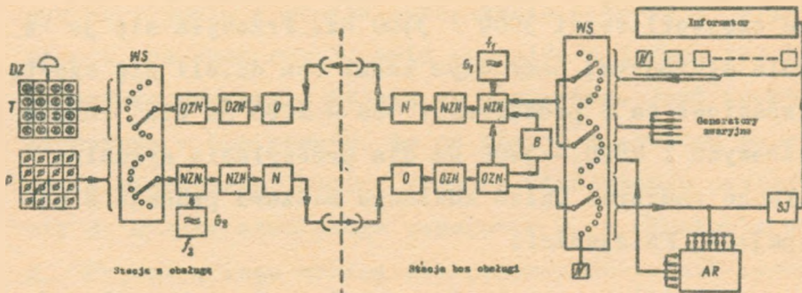
Rys. 21. Uproszczony schemat blokowy urządzeń zdalnego nadzoru linii radiowej URŁ24
