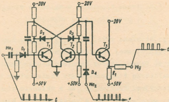
Rys. 17. Układ zamiany modulacji położenia impulsów na jednostronną modulację szerokości
