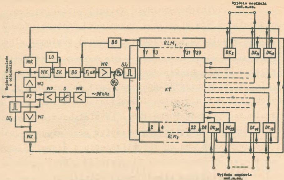
Rys. 15. Uproszczony schemat blokowy demodulatora wielokrotnego linii radiowej UR124
