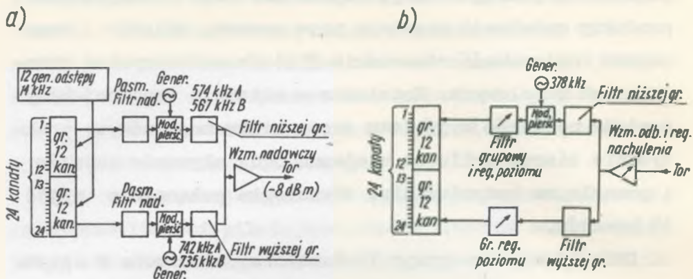
rys. 2. a/ Blokowy schemat modulatora grupowego, b/ Blokowy schemat demodulatora grupowego
