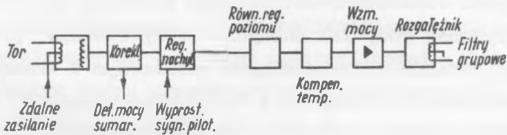
Rys. 7. Blokowy schemat wzmacniacza odbiorczego
