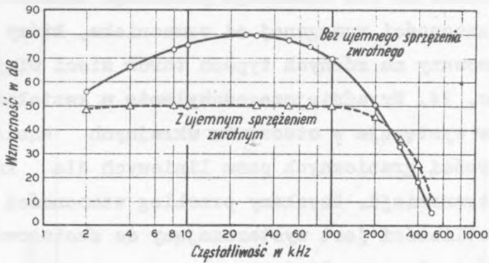
Rys. 13. Częstotliwościowa charakterystyka wzmocnienia wzmacniacza stosowanego we wzmacniaku przelotowym systemu P1
