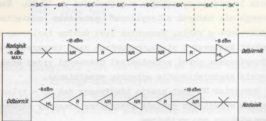
Rys. 4. Rozmieszczenie wzmacniaków
