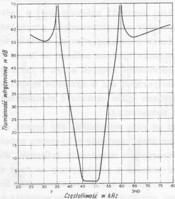
Rys. 10. Częstotliwościowa charakterystyka tłumienności wtarceniowej filtra odbiorczego.
