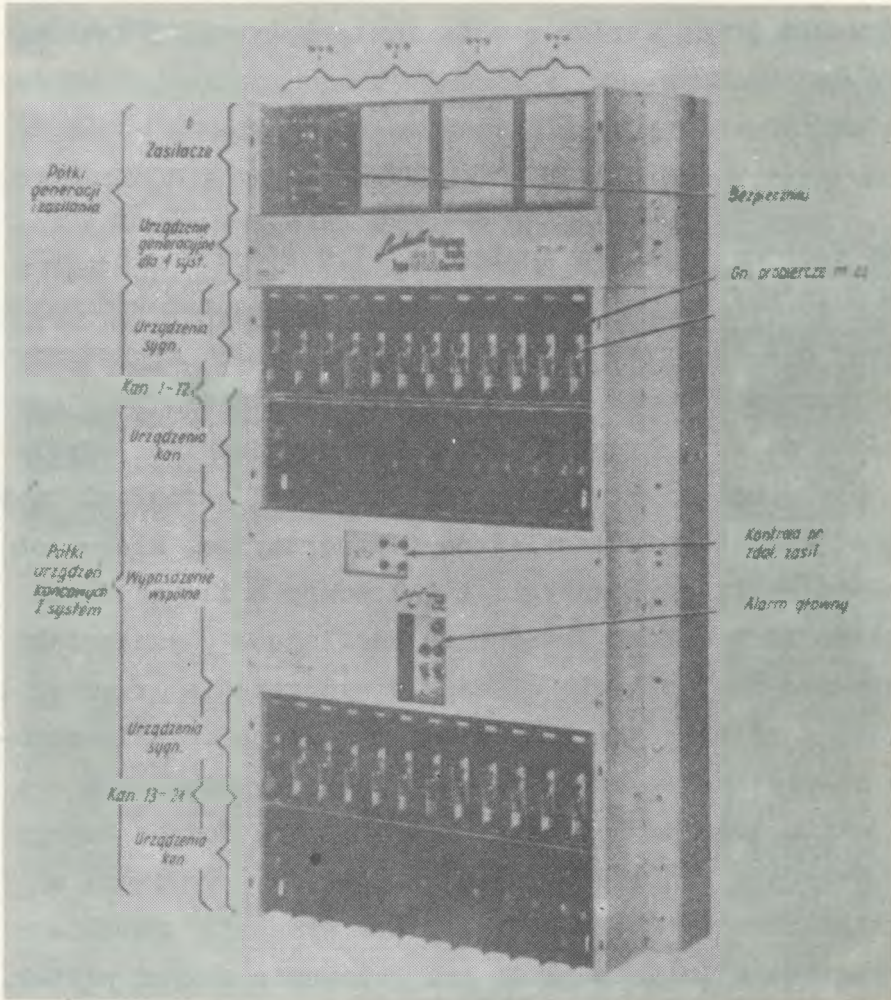
Rys. 11. Wygląd zewnętrzny stojaka urządzeń końcowych systemu SIA
