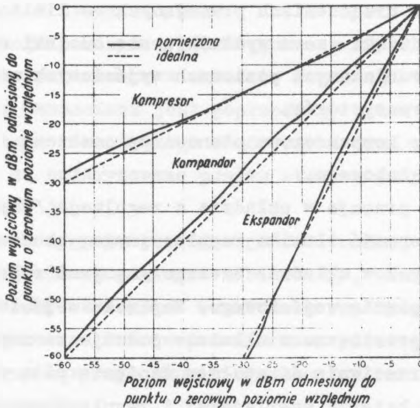
Rys. 8. Charakterystyki komparatora
