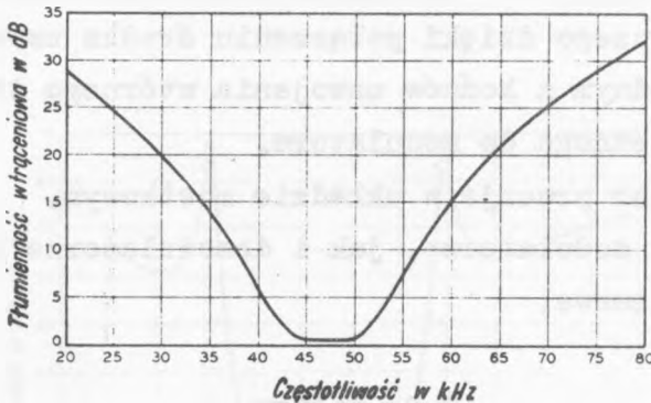
Rys. 9. Częstotliwościowa charakterystyka tłumienności wtrąceniowej filtra nadawczego
