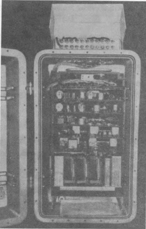
Rys. 21. Widok końcowego urządzenia abonenckiego po otwarciu pokrywy, przygotowanego do montażu na szkielet.
