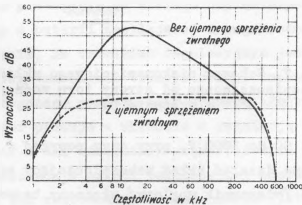
Rys. 6. Częstotliwościowa charakterystyka wzmocnienia nadawczego wzmacniacza kanałowego
