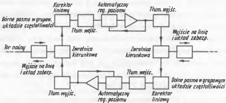
Rys. 12. Schemat blokowy wzmacniaka przelotowego
