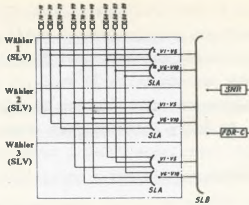
Rys. 3. Rozmieszczenie 90 linii abonenckich w wielokrociu Wähler - wybierak
