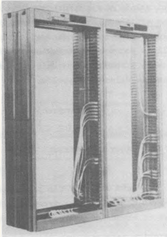
Rys. 6. Kable międzystojakowe
