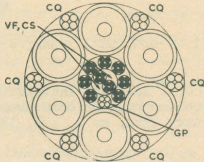
Rys. 1b). Widok poprzecznego przekroju kabla
