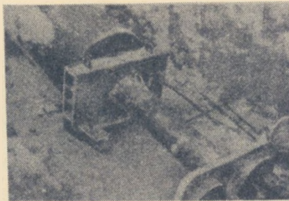
Rys. 4. Urządzenie do hydraulicznego wbijania poziomych otworów na przejścia z kanalizacją kablową
