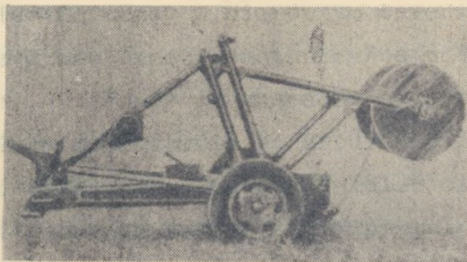
Ryc. 5. Lekki układacz kabli w czasie pracy
