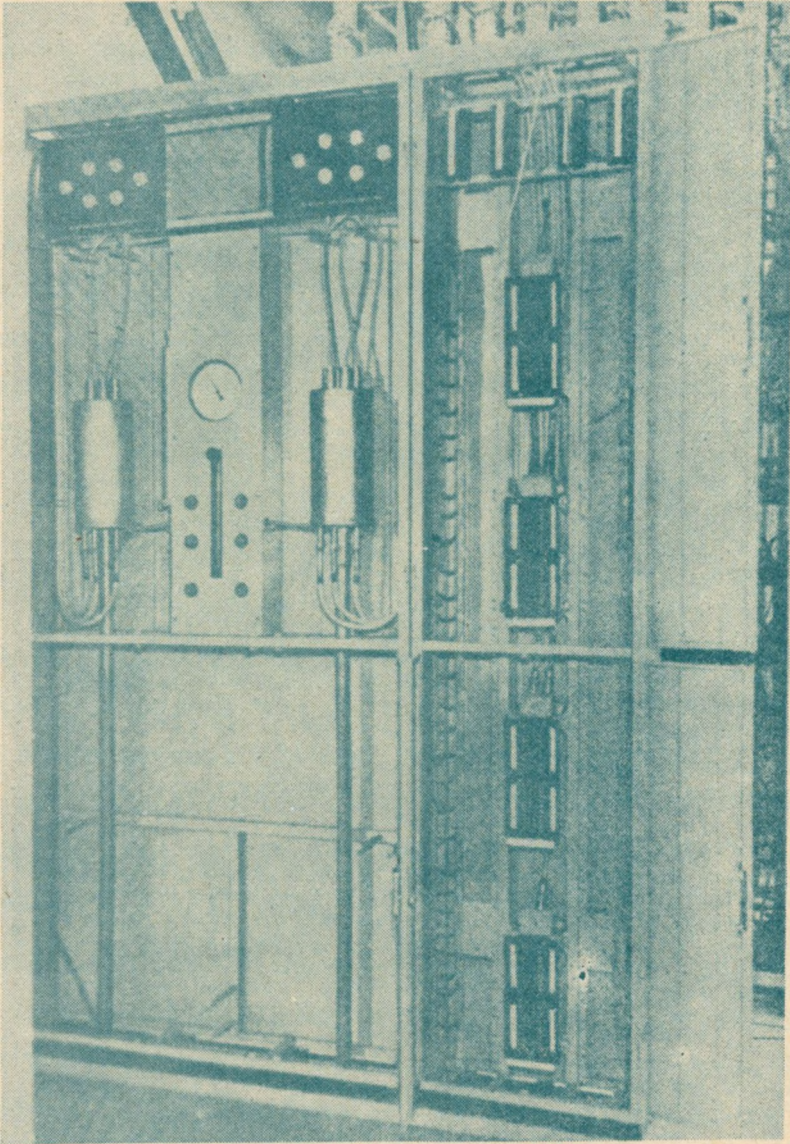
Rys. 27. Widok stojaka głowicowo-kontrolnego na głównej stacji wzmocniającej. Z lewej strony rysunku widać głowice rozdzielcze kabla współosiowego, między nimi urządzenia do kontroli ciśnieniowej kabla, z prawej strony pokazano łączówki głowic kabla symetrycznego
