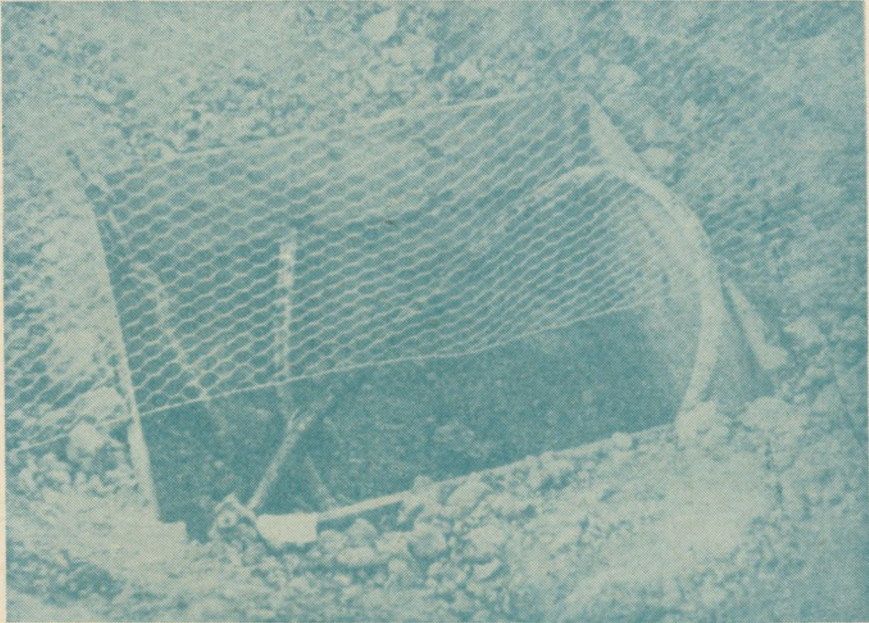
Rys. 8. Widok studni złączowej, wykonanej z desek, stosowanej pomiędzy Albury i Melbourne
