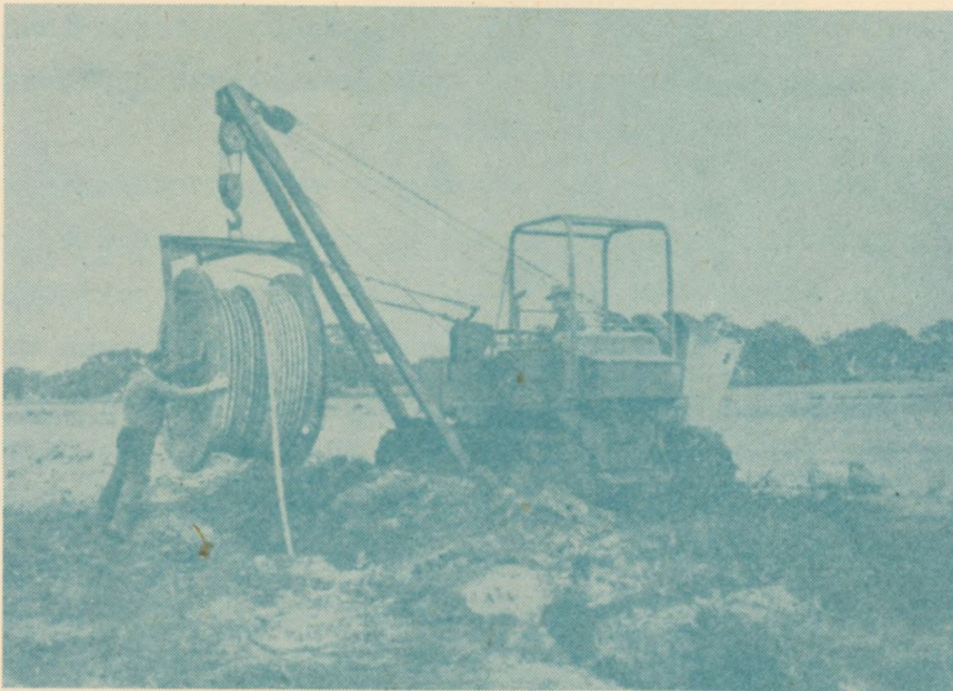
Rys. 16. Układanie kabla za pomocą ciągnika i dźwigu pokazanego na rys. 15
