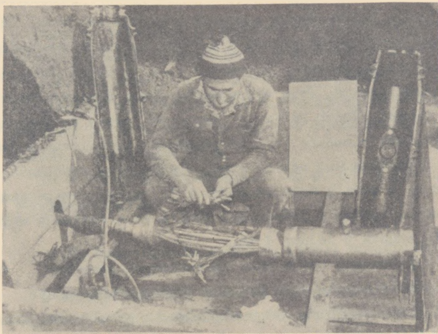
Rys. 26. Ogólny widok na wnętrzu studni złączowej. Z prawej strony rysunku widać na kablu osłonę miedzianą, przy złączu końcówki nasadkowe a z obu stron kablarza połówki mufy żeliwnej
