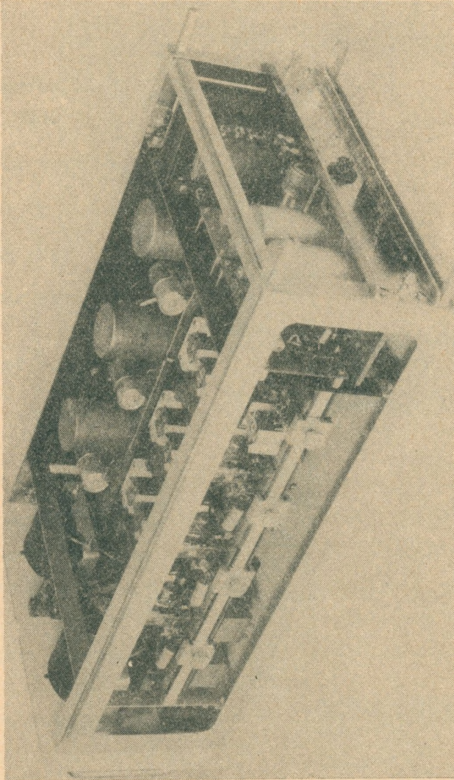
Rys. 2. Widok stereodekodaera pomiarowego po zdjeciu obudowy
