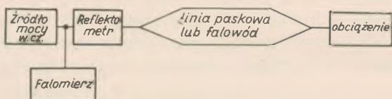
Rys. 16. Zestaw do wzorcowania mierników PEM w przewodnicy falowej
