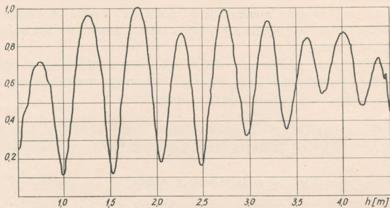
Rys. 2. Rozkład przestrzenny fali stojącej; polaryzacja pionowa; podłoże suche
