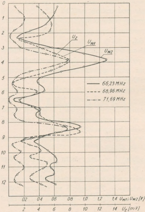
Rys. 6. Rozkład fali stojącej wzdłuż masztu — warunki rzeczywiste
