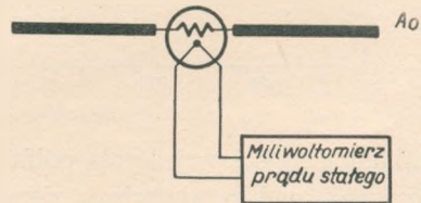
Rys. 11. Pomiar prądu we wzorcowej antenie odbiorczej
