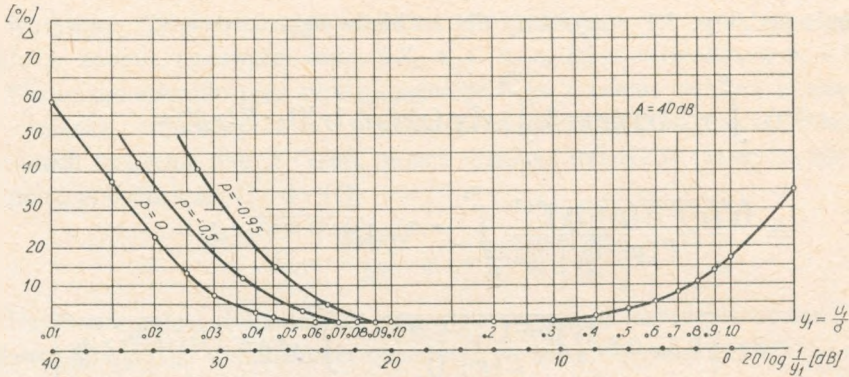
Rys. 5. Charakterystyki błęd pomiaru \Delta mocy średniej sygnału o rozkładzie typu \Gamma w funkcji dolnej granicy przetwarzania y_1 dla różnych wartości parametru p i ustalonej wartości dynamiki A = 40 dB
