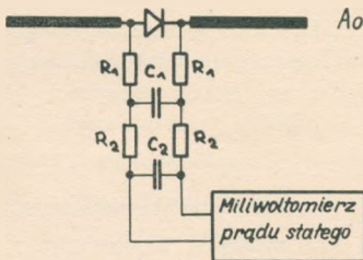
Rys. 10. Pomiar SEM we wzorcowej antenie odbiorczej
