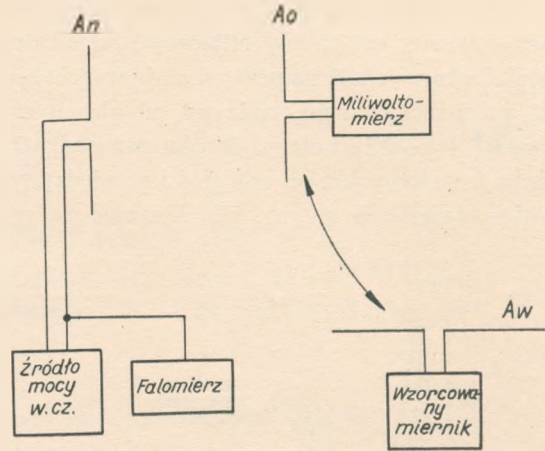
Rys. 9. Wzorcowanie miernika PEM z anteną dipolową metodą wzorcowej anteny odbiorczej (widok z góry)
