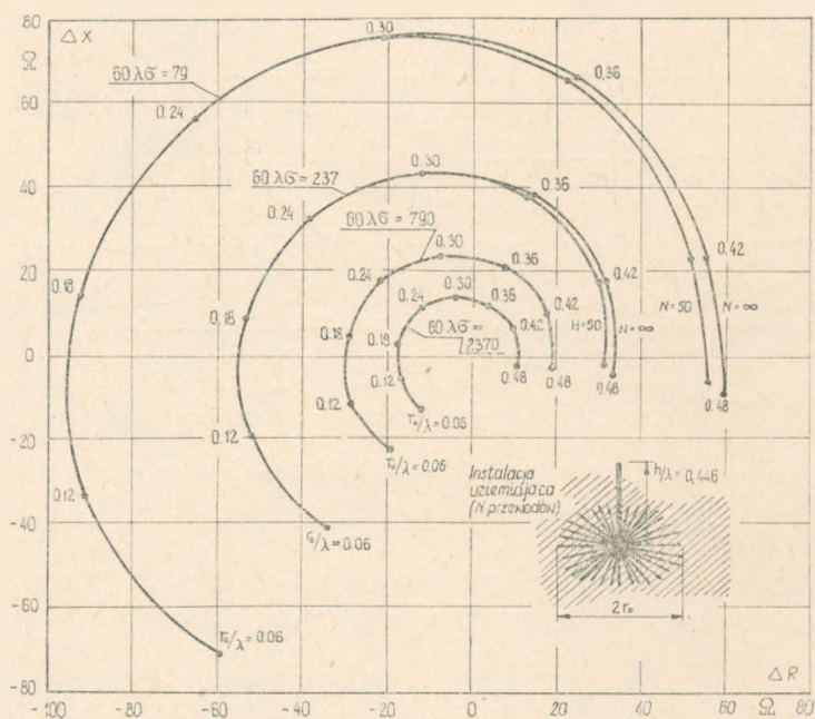
Rys. 12. Zależność zmian impedancji wejściowej anteny od promienia instalacji uziemiającej i konduktywności ziemi
