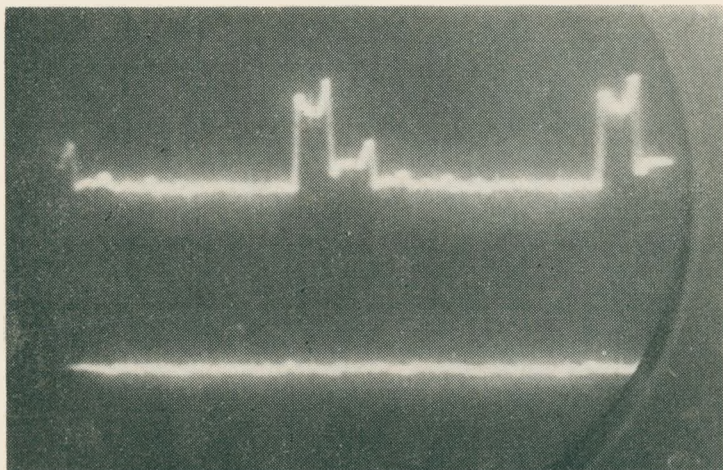
Rys. 3. Przebiegi w układzie koder (punkt A) i dekodera (punkt B) dla sygnału czerni (000000)
