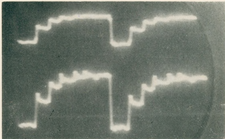
Rys. 2. Przebiegi w układzie koder (punkt A) i dekodera (punkt B) dla sygnału bieli (111111)
