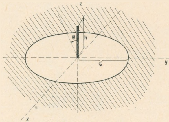
Rys. D-1. Antena nad instalacją uziemiającą w postaci metalowego dysku
