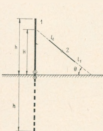
Rys. 17. Dwa odcinki linii odciągowej tworzą antenę bierną umieszczoną w polu bliskim anteny czynnej (masztu)
