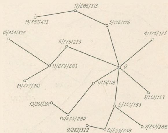
Rys. 8. Konfiguracja sieci 17-to węzłowej przy ograniczeniu wydłużenia dróg transmisji do K < 1,26 . Sumaryczna długość sieci D = 2282 km. Maksymalne wydłużenie drogi transmisji K_{max} = 1,26
