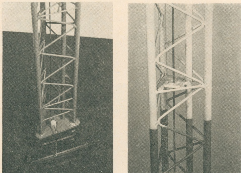
Rys. 43. Fragmenty modelu anteny w skali 1:40
