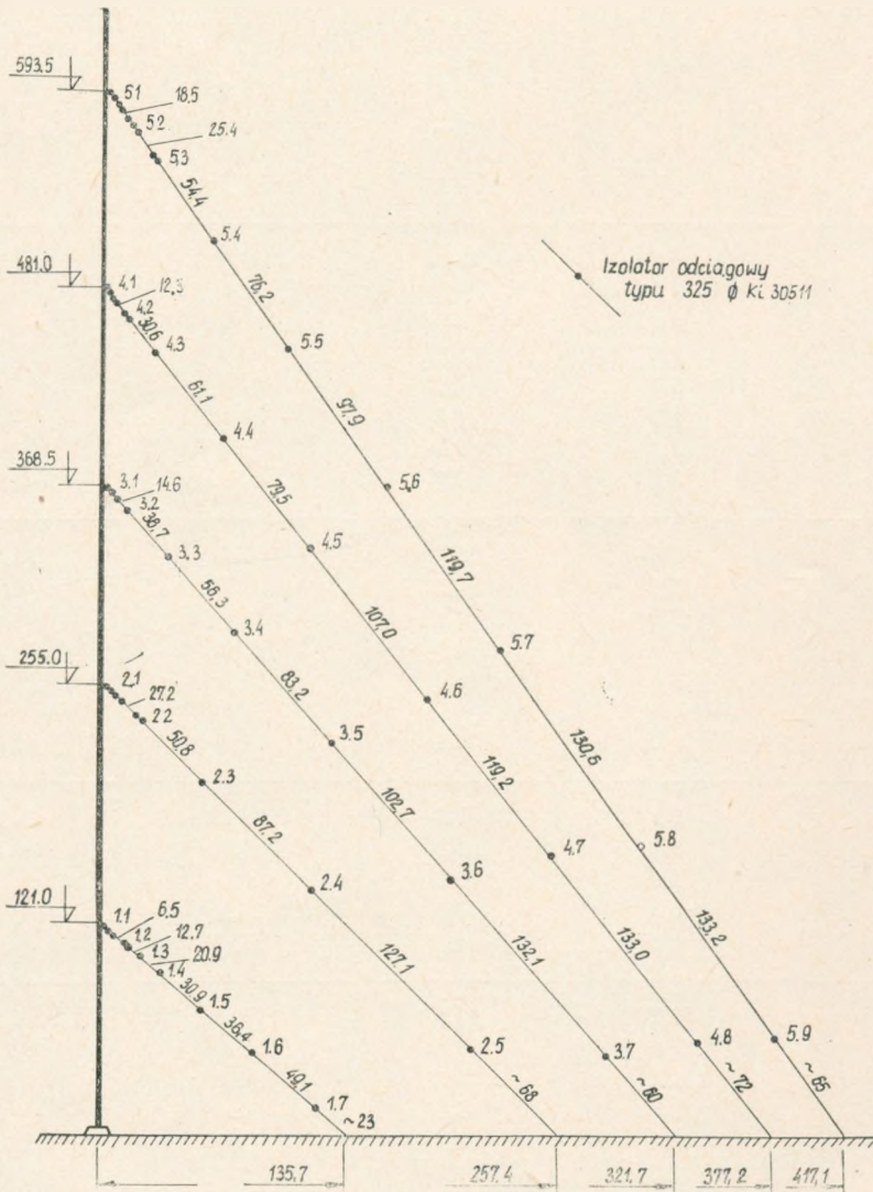
Rys. 24. Rozmieszczenie izolatorów odciągowych
