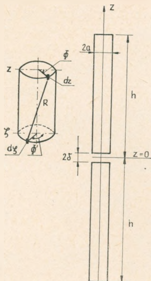
Rys. 4. Symetryczna antena cylindryczna
