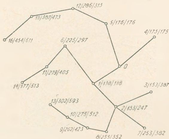
Rys. 5. Konfiguracja sieci 17-to węzłowej bez ograniczenia wydłużenia dróg transmisji K < \infty Maksymalne wydłużenie drogi transmisji K_{\max} = 2,53 Sumaryczna długość sieci D = 2049 km
