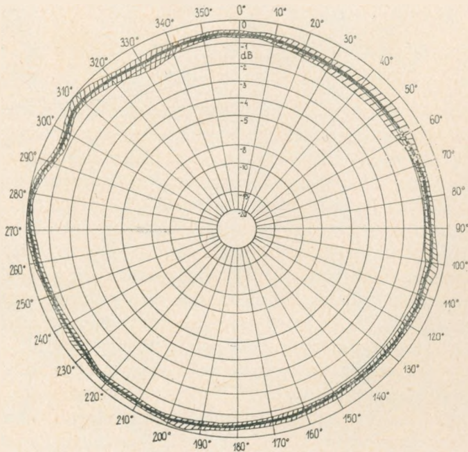
Rys. 51. Charakterystyka promieniowania w płaszczyźnie poziomej anteny WRC [hatched] – rozrzut wyników pomiarów, ——— — charakterystyka uśredniona
