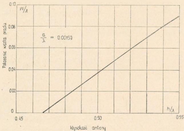
Rys. 6. Położenie węzła prądu na antenie cylindrycznej w funkcji jej wysokości
