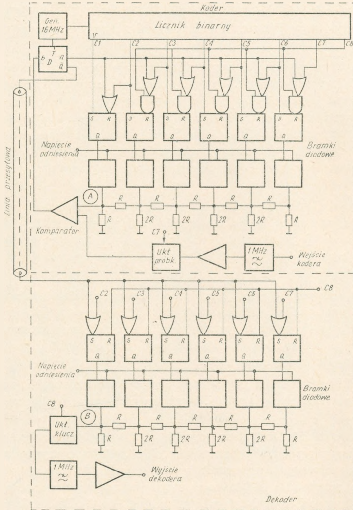
Rys. 1. Schemat blokowy kodera i dekodera wizjotelefonicznego
