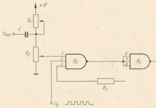
Rys. 1. Schemat blokowy komparatora
