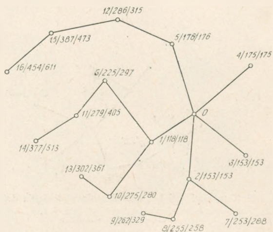
Rys. 7. Konfiguracja sieci 17-to węzłowej przy ograniczeniu wydłużenia dróg transmisji do K < 1,58 . Sumaryczna długość sieci D = 2159 km. Maksymalne wydłużenie drogi transmisji K_{max} = 1,45
