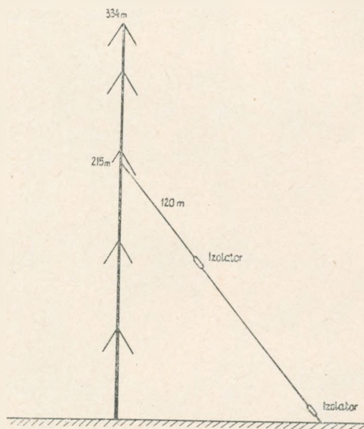
Rys. 28. Sposób zawieszenia i izolacji odciążu pomiarowego
