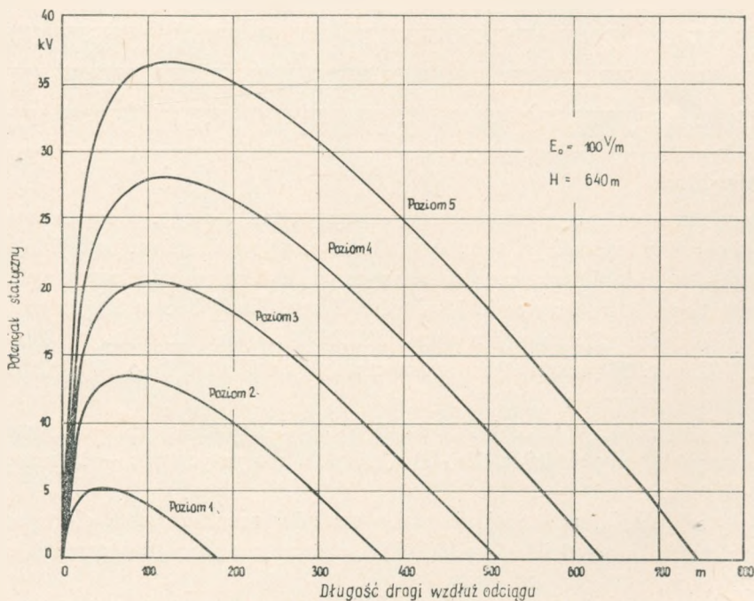
Rys. 23. Rozkład potencjału statycznego wzdłuż drogi odcinków ( E_0 = 100 \text{ V/m} )
