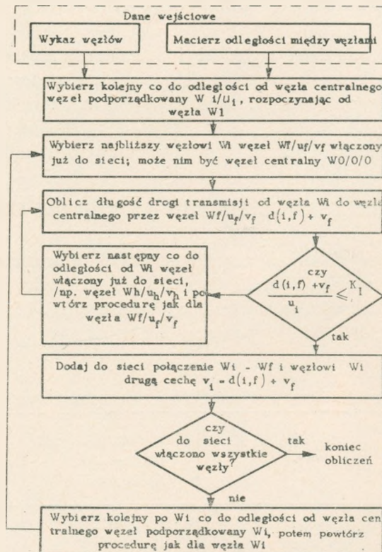
Rys. 4. Schemat (algorytm) konstruowania sieci rozsiewczej
